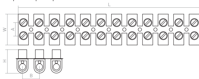
Габаритные размеры
